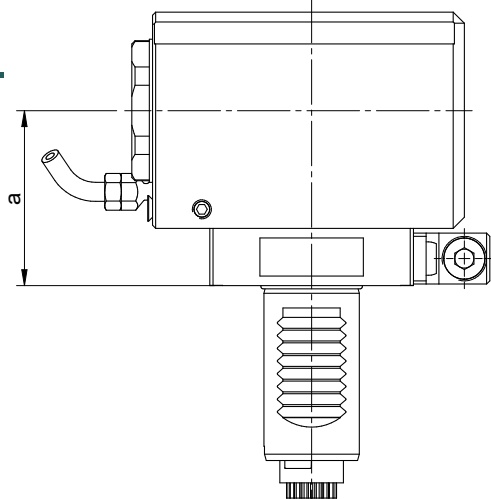
內牙款式 - Internal Nut type
